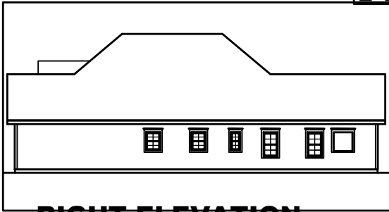
RIGHT ELEVATION
