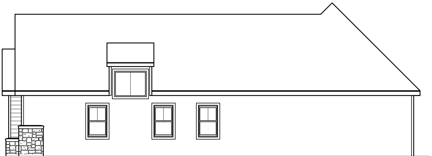
RIGHT ELEVATION
