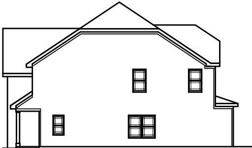
RIGHT ELEVATION
